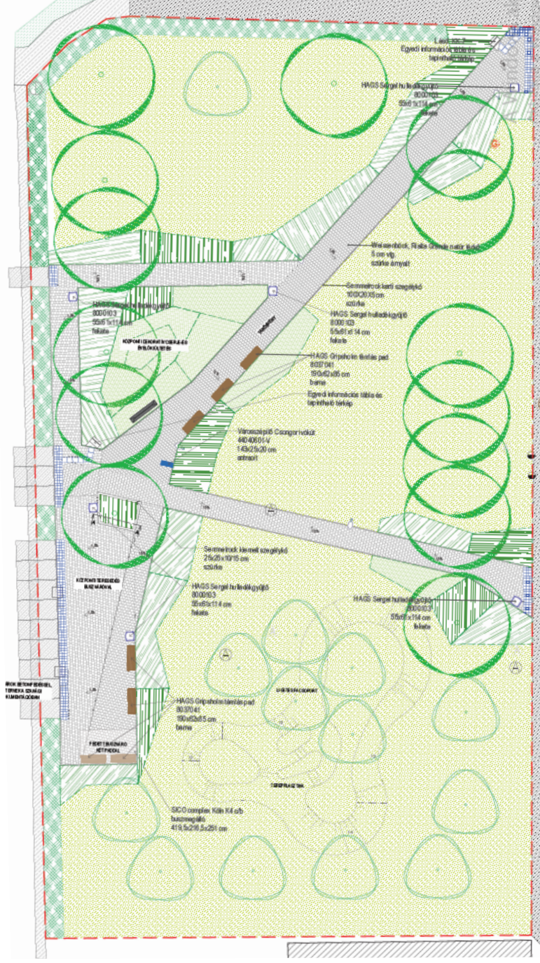
Vasútállomás mellett park felülnézet (Forrás: S-TÉR Kft. kivitelei tervdokumentáció részlet)
